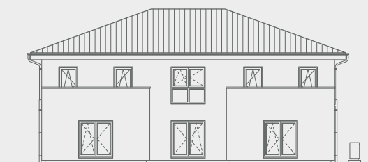
Ansicht Hinten
