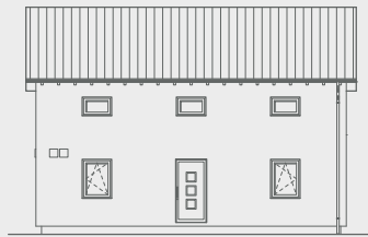
Ansicht Eingang
