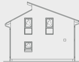
Ansicht Links
