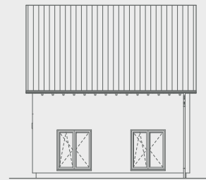
Ansicht Hinten
